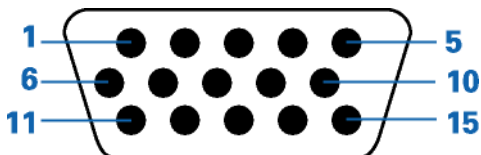
15 ピンカラーディスプレイ信号ケーブル
