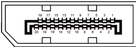
20-poliges Farbdisplay-Signalkabel
