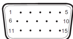
Καλώδιο σήματος έγχρωμης οθόνης 15 ακίδων
